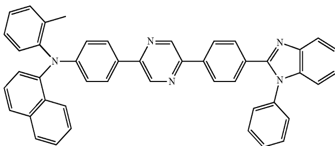
N-(4-(5-(4-(1-phenyl-1H-benzo[d]imidazol-2-yl)phenyl)pyrazin-2-yl)phenyl)-N-(o-tolyl)naphthalen-1-amine
