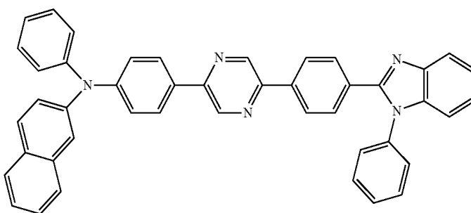
N-phenyl-N-(4-(5-(4-(1-phenyl-1H-benzo[d]imidazol-2-yl)phenyl)pyrazin-2-yl)phenyl)naphthalen-2-amine
